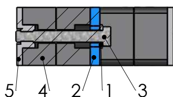
SCHNITT D-D MAßSTAB 1 : 2
