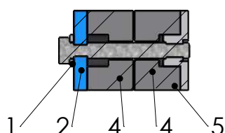
SCHNITT C-C MAßSTAB 1 : 2
