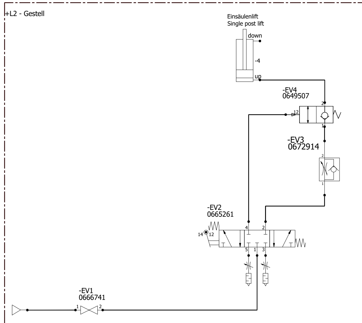
Einsäulenlift stationär 3750N Single post lift stationary 3750N
